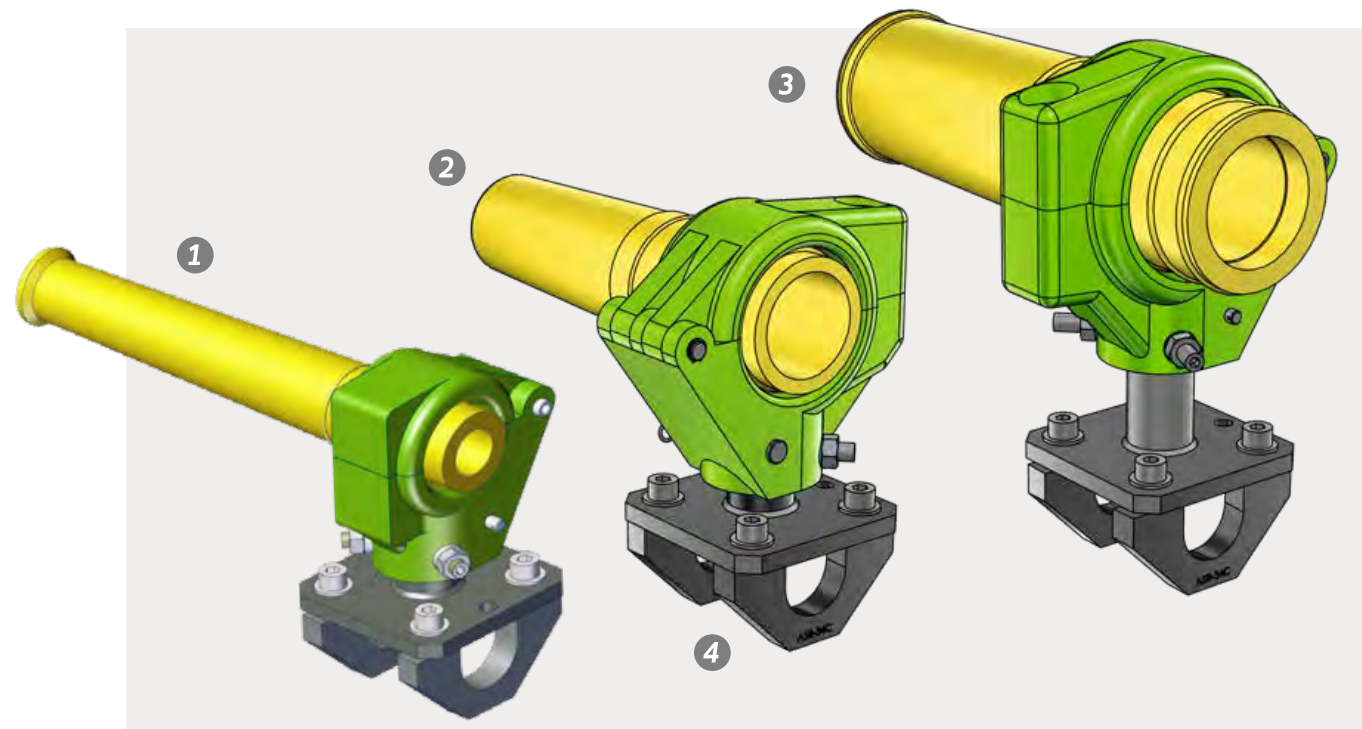
上述组件示例展示了黄色旋转杆、相应的支架、金属支架，以及适配 Ø 34mm 管子的管夹。
