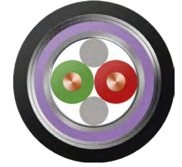
PROFIBUS DP
