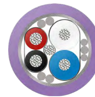
DeviceNet™
