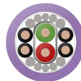
PROFIBUS DP-Desina
