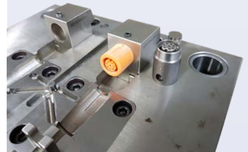
Abbildung 2: 3D-gedruckte Aufnahme in einem Werkzeug
